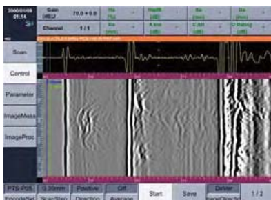
Raw TOFD Image
